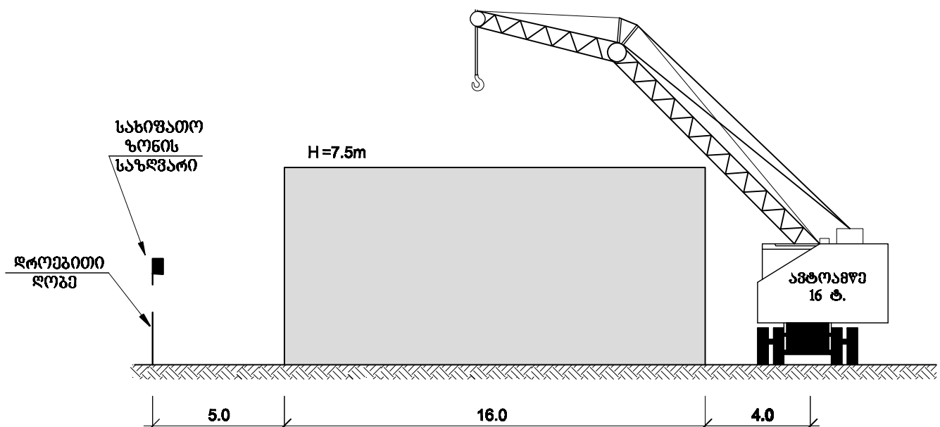
სადემონტაჟო სქემა
